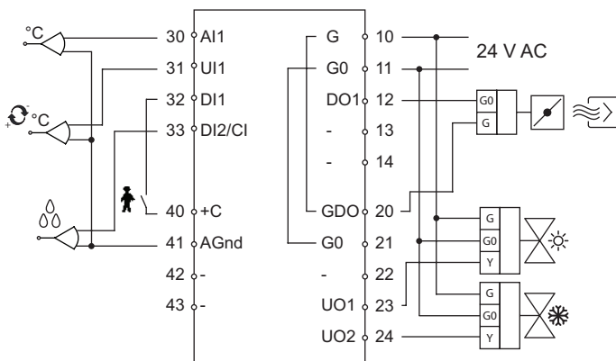
Figur 4. Inkopplingschema för RC-H
