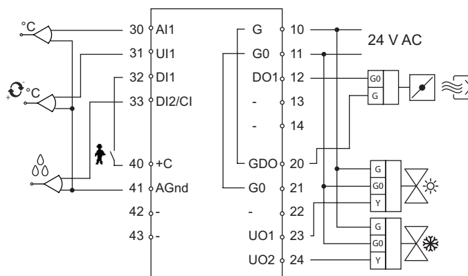
Abb. 4. Anschlussplan für RC-H
