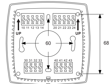
Figure 3. Socle et emplacement des bornes de connexion (dimensions en mm).
