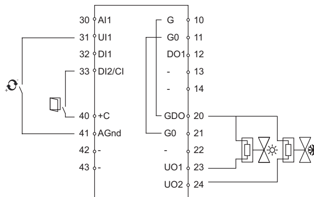
Figur 5. Alternativt inkoppling för plint 31, UI1, plint 33, DI2/CI, plint 23, UO1, och plint 24, UO2.
