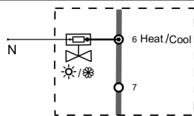
Fig. 2 Cablaggio due tubazioni
