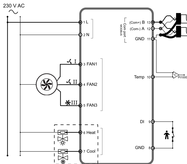
Fig. 1 Cablaggio quattro tubazioni
